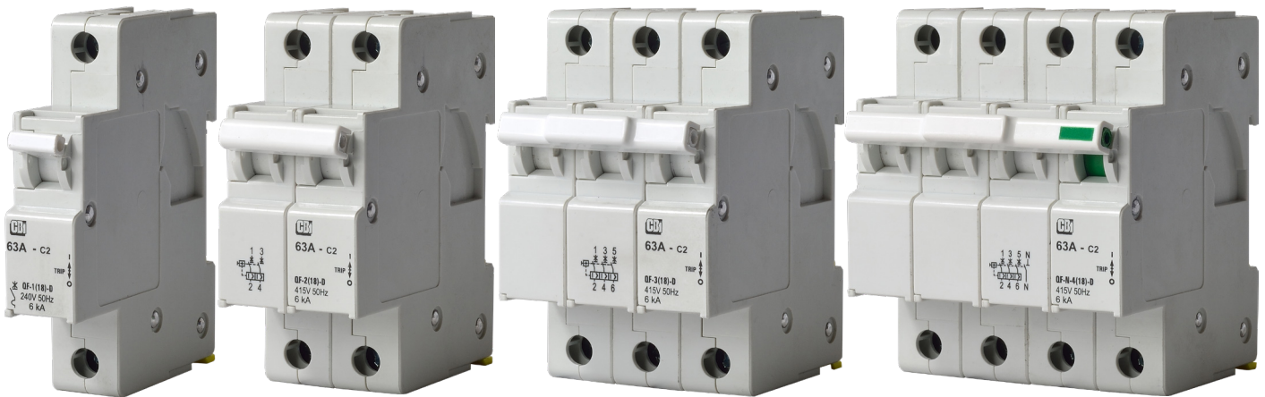
1 pole DIN Mount
